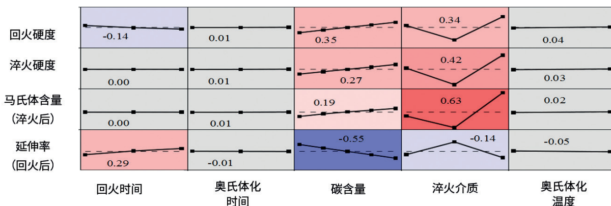
主效应矩阵图——结果的统计学评估
