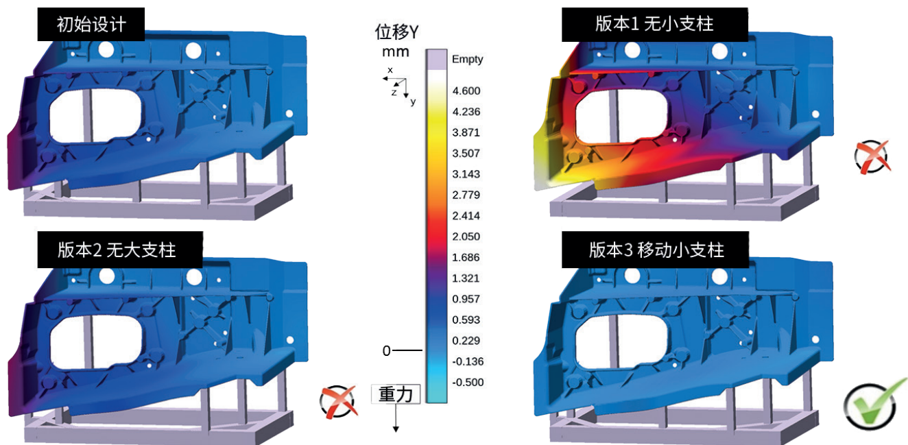
评估不同的热处理支架设计
