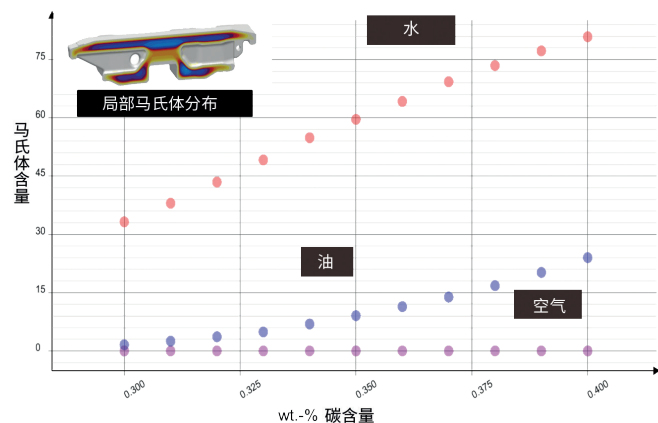
马氏体含量与碳含量和淬火介质的关系
