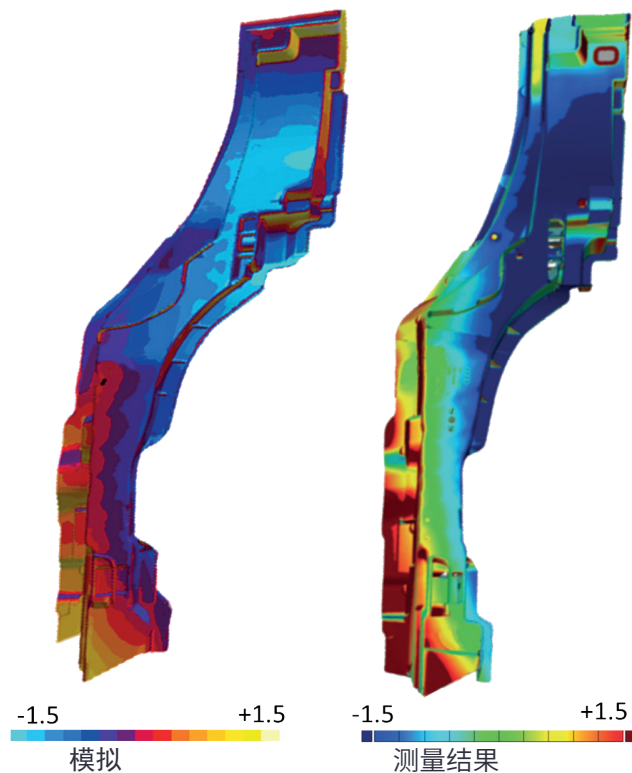
使用6点方法评估预测的变形
