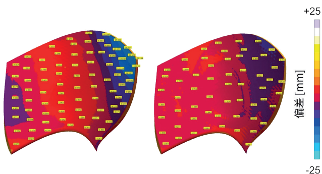
整个工艺过程结束后，与原始形状(左)相比，使用模具中的预补偿减少了变形
