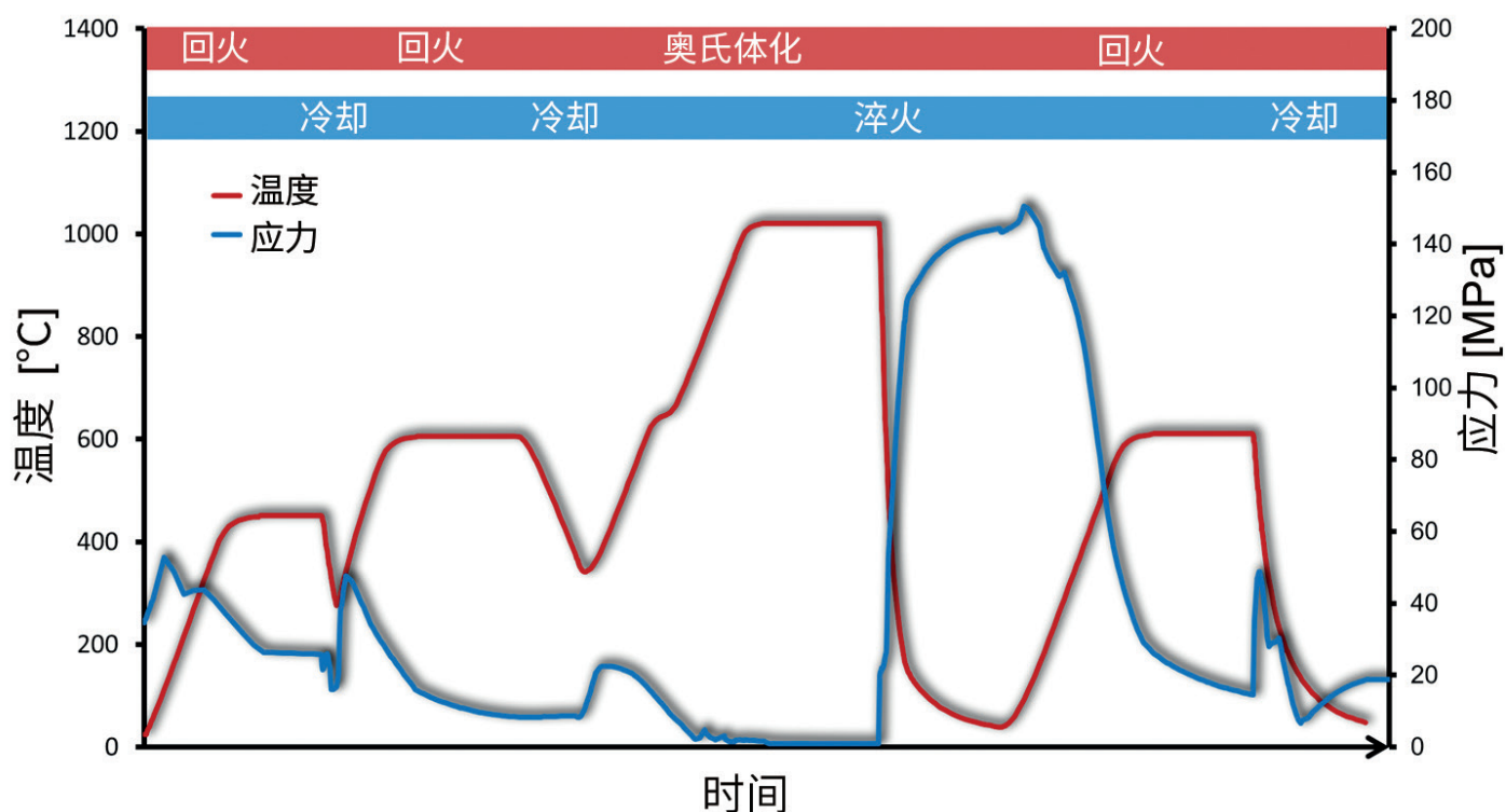
热处理过程中的温度曲线和相关应力变化
