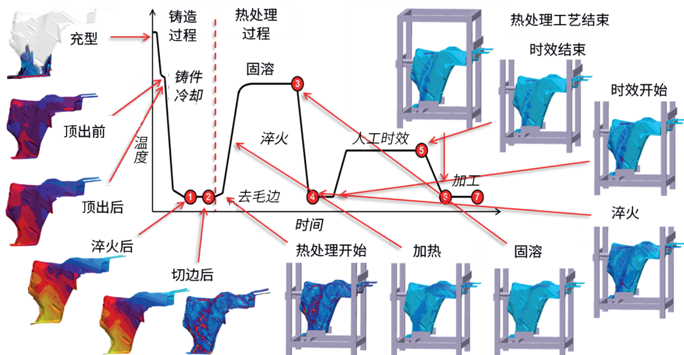
铸造和热处理工艺过程的集成建模
